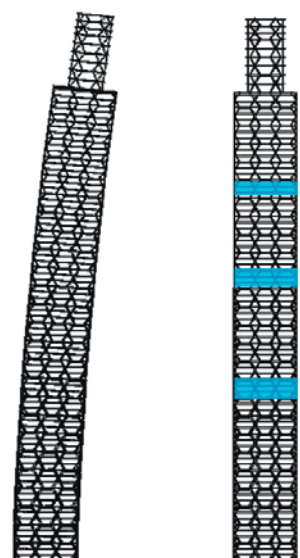
Рис. 5. Поперечное смещение конструкции под воздействием ветра
