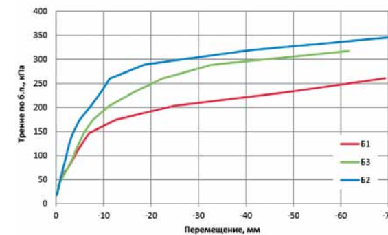
Рис. 22. Величина удельного трения по боковой поверхности средней части баретты в зависимости от перемещения
