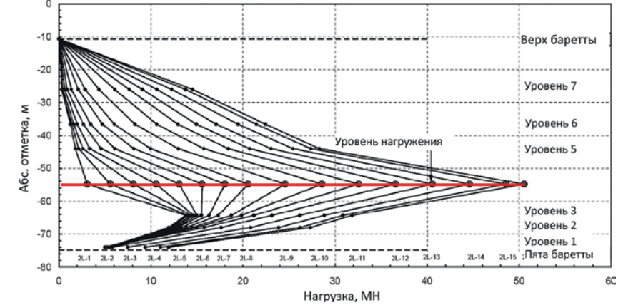
Рис. 23. Распределение усилий, действующих по глубине баретты Б1 при нагружении нижнего уровня домкратов
