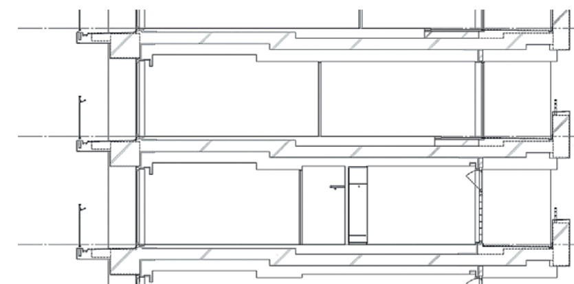
Разрез жилой зоны
