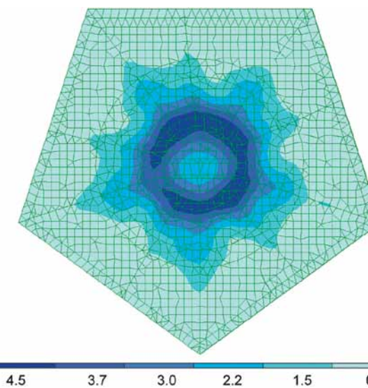
Рис. 2. Безразмерная схема распределения нагрузки, передаваемой на фундамент башни. Нагрузка показана в долях от средней равномерно распределенной нагрузки
