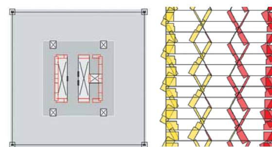
Рис. 8. Анализ осевой нагрузки под действием нормального давления/ветра
