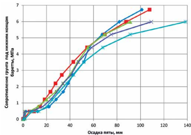
Рис. 18. Зависимость сопротивления по пяте баретты от перемещения
