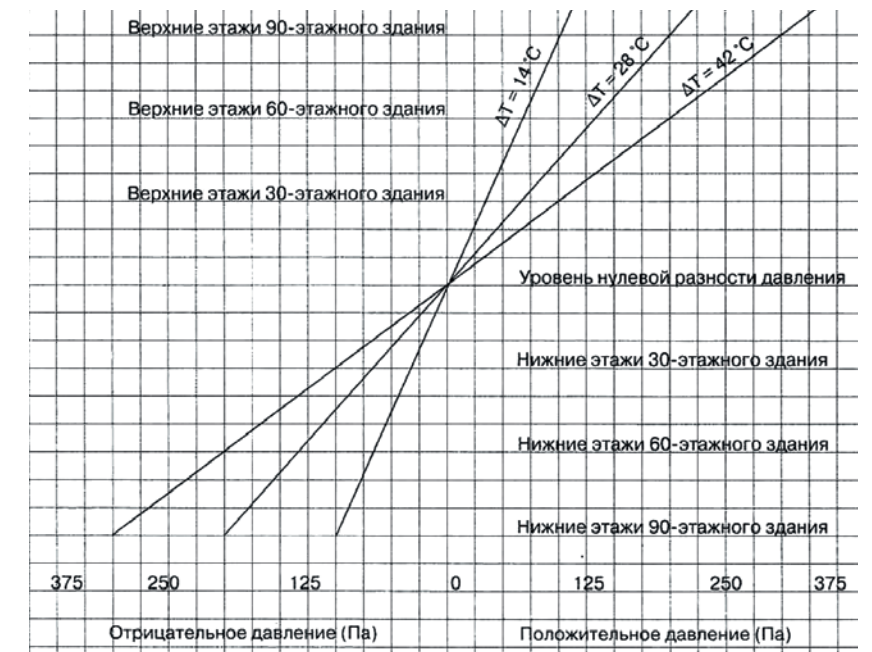
Рис. 7. Теоретический градиент давлений для различных значений высоты здания и разности температуры воздуха
