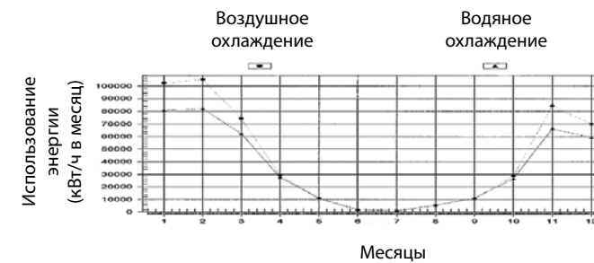
Рис. 5. Использование электрической энергии по месяцам. Входные данные
