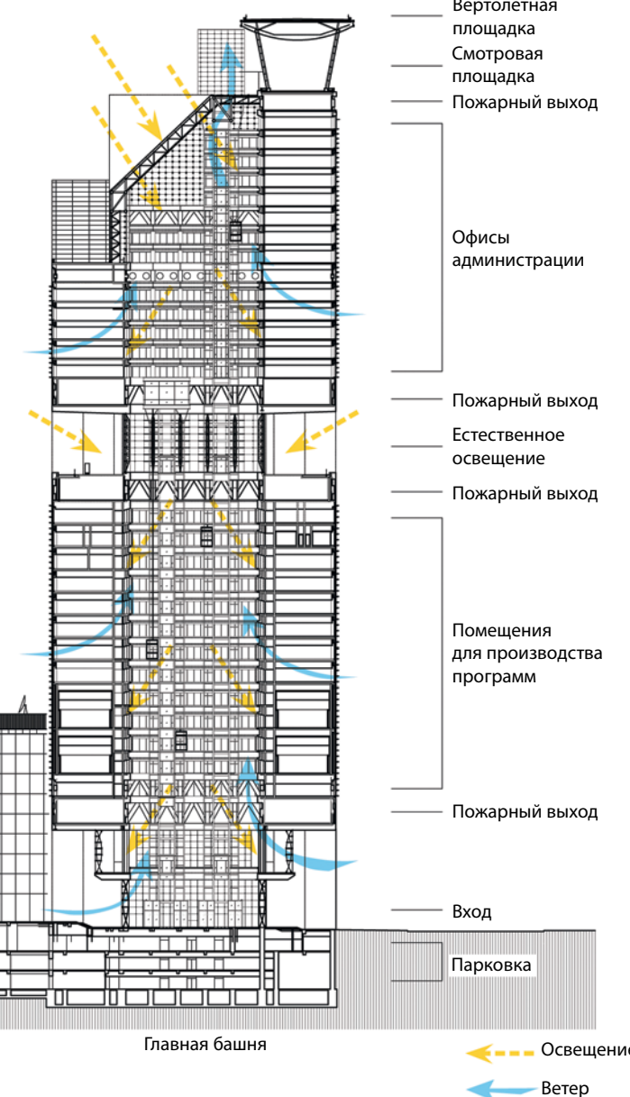
Вертикальный разрез здания
