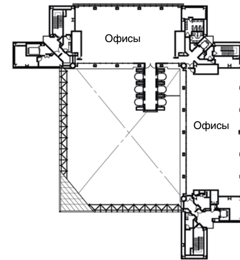
План 33 этажа
